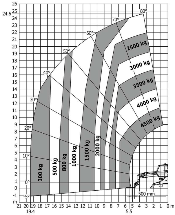
フォークアウトリガー使用 (TFF5T)Ref.931267
