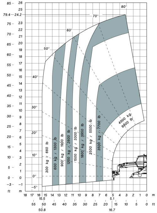
ウィンチ(Winch5T) Ref.921341
