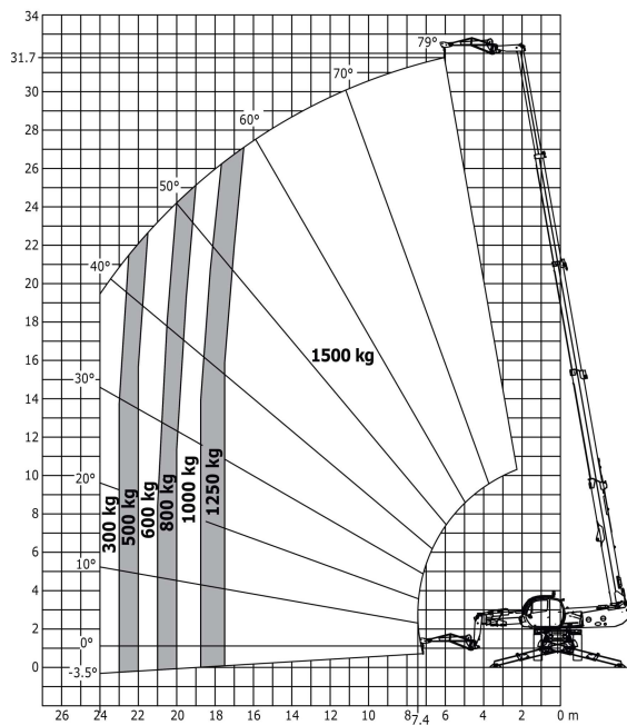
ジブ(PT1500) Ref.921330
