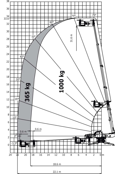
高所作業車(PSE4400/1000D) Ref.939500
