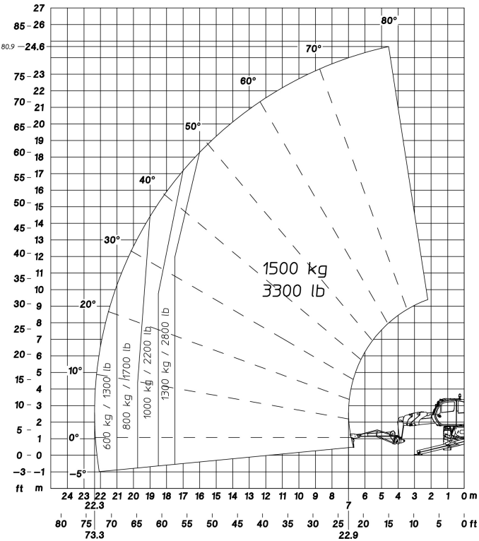
延長ジブ (P1500) Ref.921319
