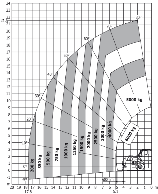
フォーク (TFF5t) Ref.53027273
