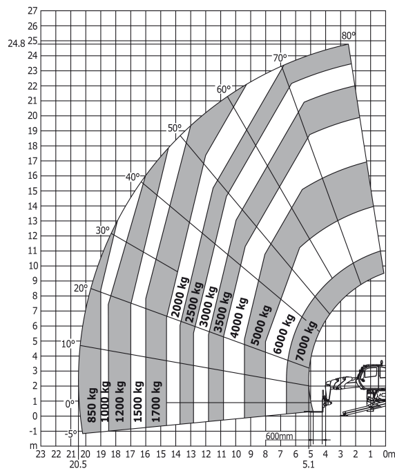
アウトリガー使用時フォーク(TFF7t) Ref.53022260
