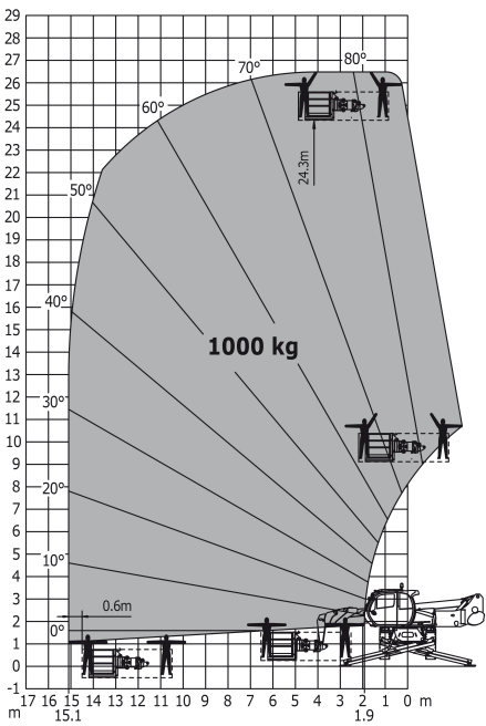
高所作業車用 Gondola (PSE4400/1000D) Ref.939500
