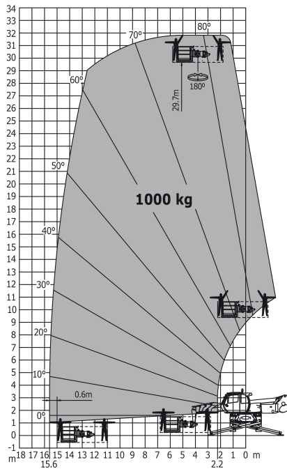
高所作業車用 Gondola (PSE4400/1000D) Ref.939500
