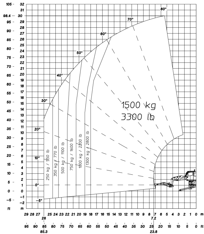
ジブ (P1500) Ref.921319
