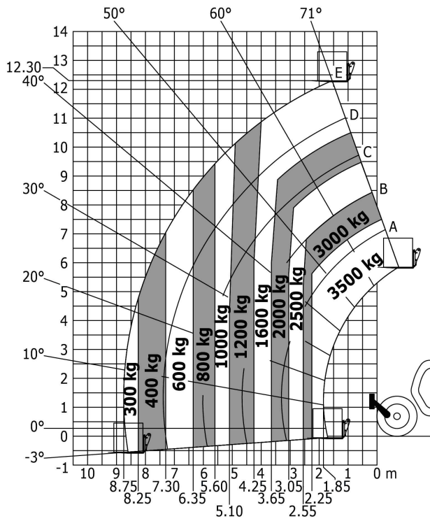
フォーク(TFF35MT) アウトリガー未使用時 Ref.788793
