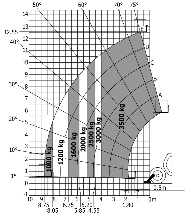
フォーク(TFF35MT) アウトリガー使用時 Ref.788793
