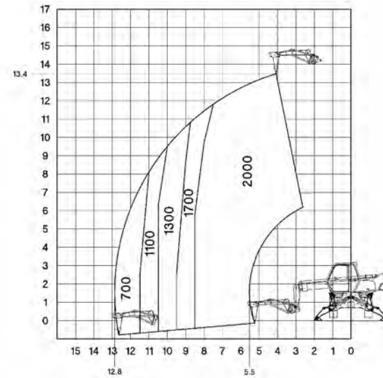
ウインチ付延長ジブ(PT2000)
