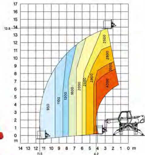
フォークアウトリガー使用時
