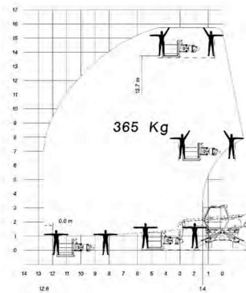
高所作業用ゴンドラ(PSE400 3650)
