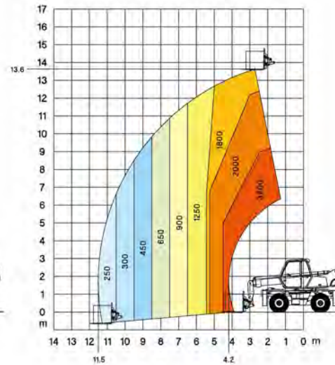
フォークアウトリガー未使用時
