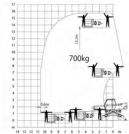
高所作業用ゴンドラ(PSE4400-700D)
