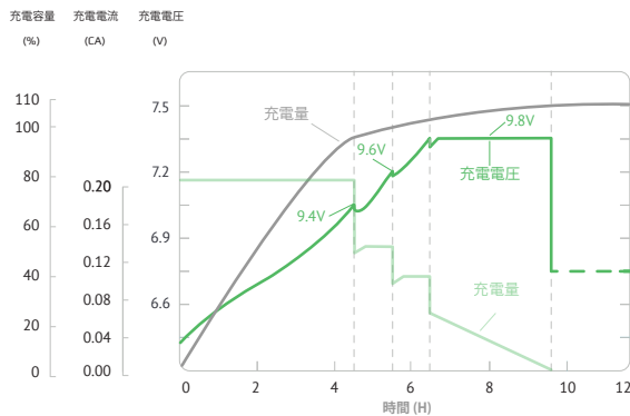
レギュラーサイクル充電特性 25°C (77°F).
