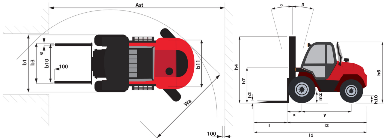
M 50-4 ST5 - 寸法図
