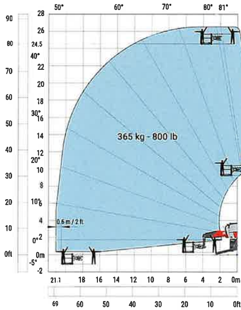
スタビライザー使用時 365kgアクセスプラットフォーム - メートル法
