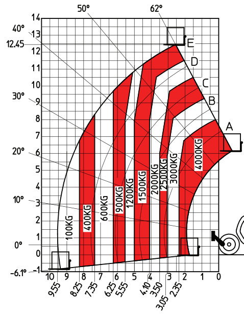
フォークアウトリガー未使用時
