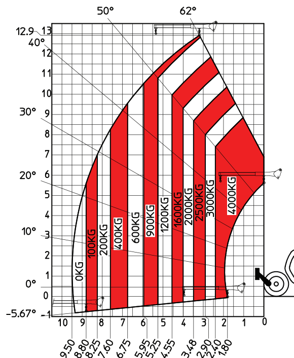
延長ジブ (P 4000) アウトリガー未使用時
