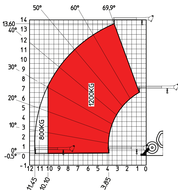
延長ジブ (P 4000) アウトリガー使用時
