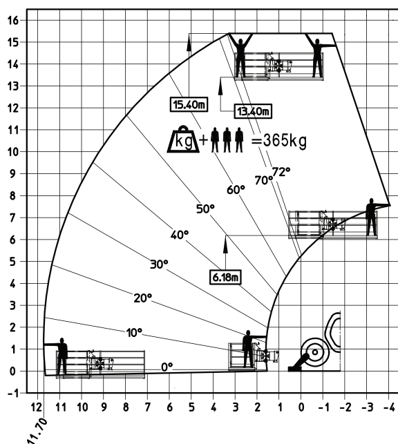
高所作業車用ゴンドラ (PSE 4400/365 D)
