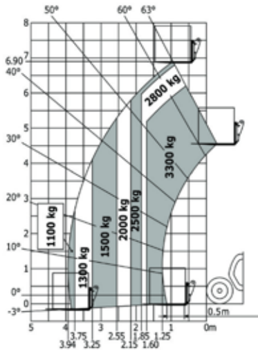
MT733EASY
