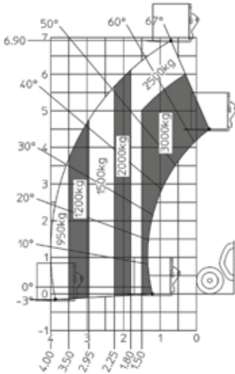
MT733EASY
