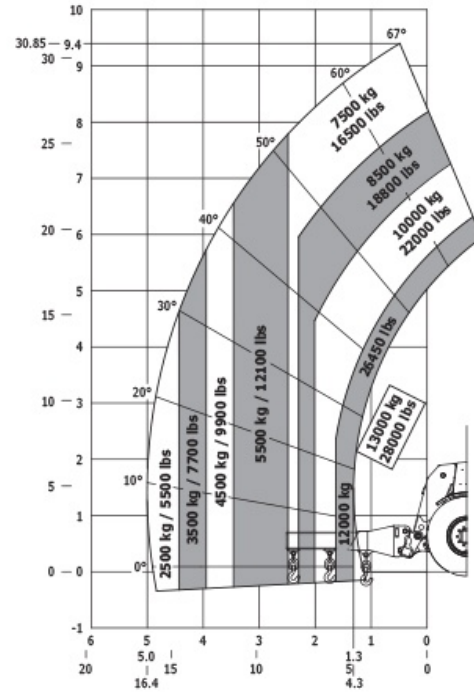
ジブ P13T Ref.53009841
