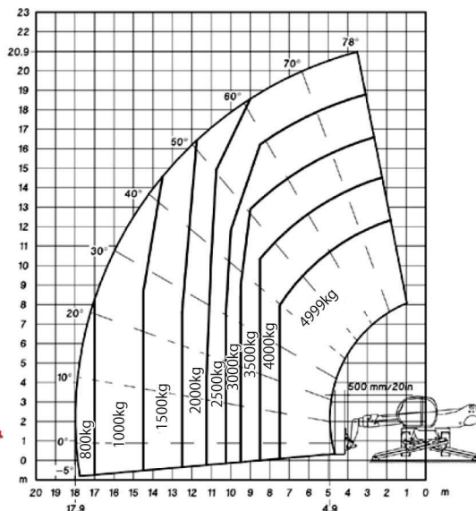
フォークアウトリガー使用時
